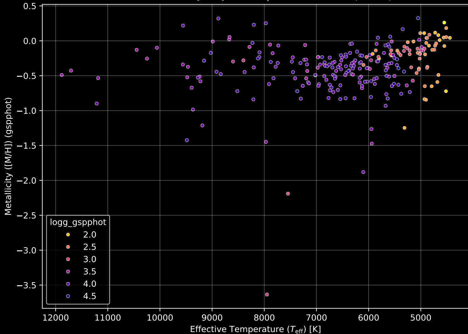
GALAH DR4 Field: [8684] Stellar Population Parameters (n= 253)
