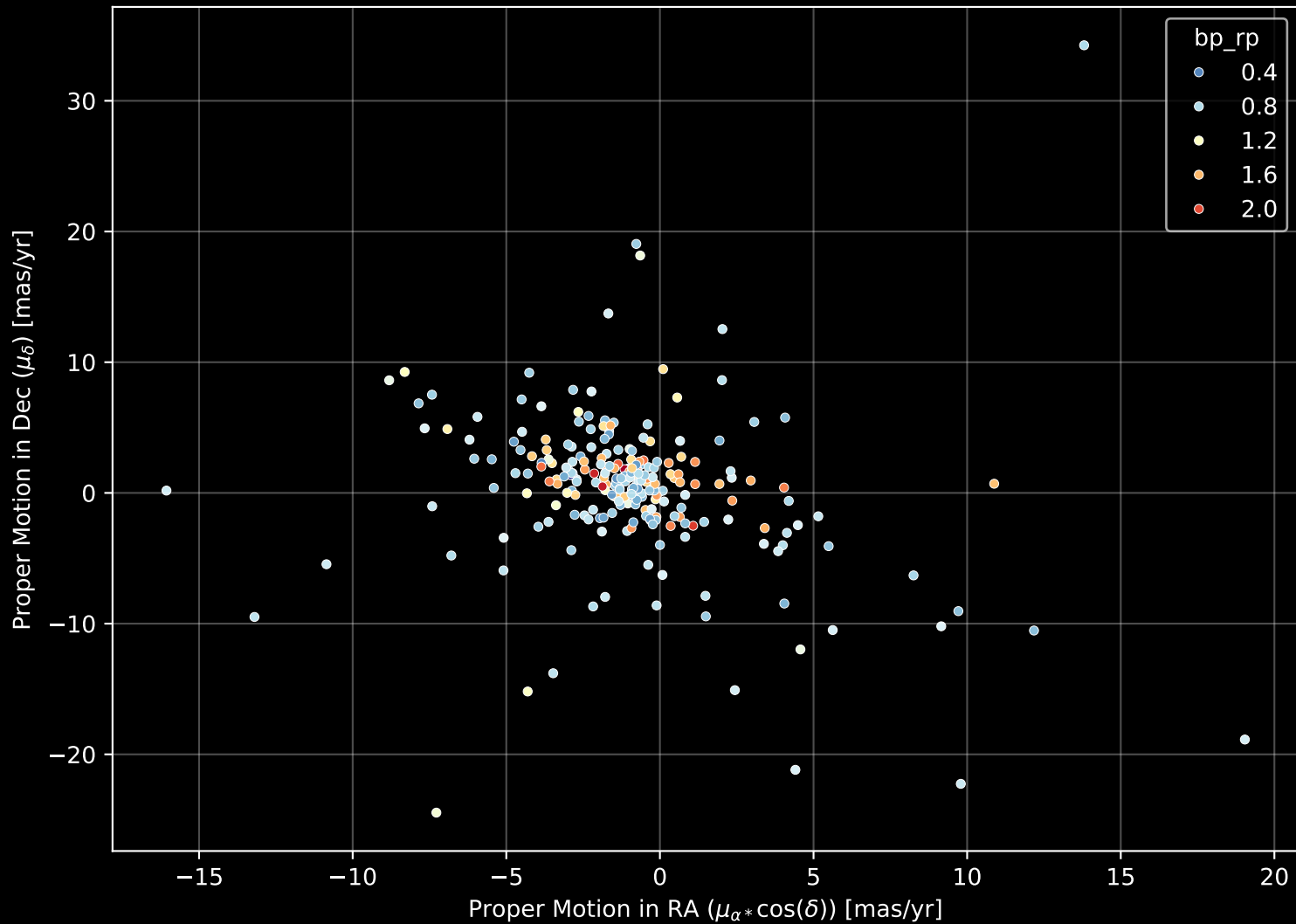
GALAH DR4 Field: [8684] Proper Motion Diagram (n= 253)
