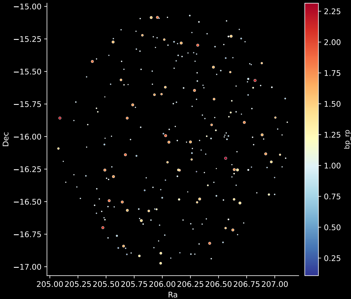
GALAH DR4 Field: [8684] Stars: 253
