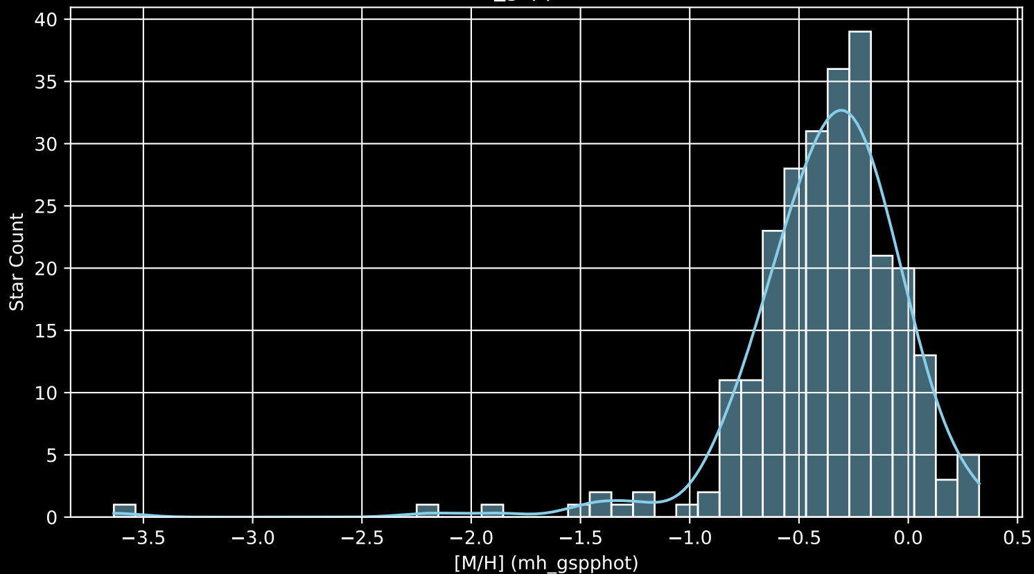
GALAH DR4 Field: [8684] [M/H] (mh_gspphot) (n= 253)
