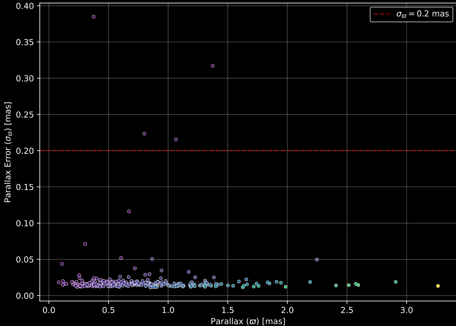
GALAH DR4 Field: [8684] Parallax Quality (n= 253)
